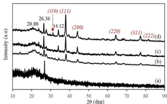
Fig. 8: The X-ray diffractograms of (a) natural diatomite, (b) AgNp-1%-NDs-Calc, (c) AgNp-3%-NDs-Calc, and (d) AgNp-5%-NDs-Calc
