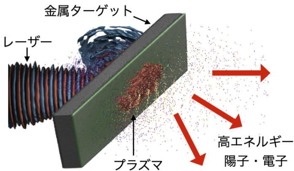
図1：超高強度レーザーによる粒子加速のシミュレーション。レーザーは図の左から灰色で示された金属ターゲットに照射され、ターゲット上に赤で示された強い加速電場が誘起される。この加速電場によって、ターゲット表面の陽子などの粒子が、高エネルギーに加速される。
