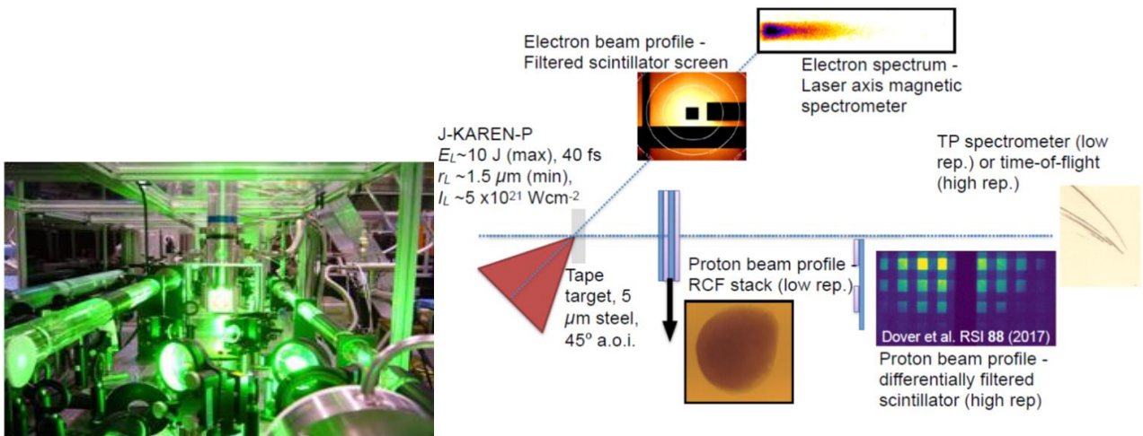
図 2：世界最高強度を誇る関西研の J-KAREN レーザーシステム（左）と実験のセットアップ（右）。J-KAREN レーザーがターゲットに照射され発生する電子及び陽子のエネルギースペクトルと空間分布を同時に計測した。
