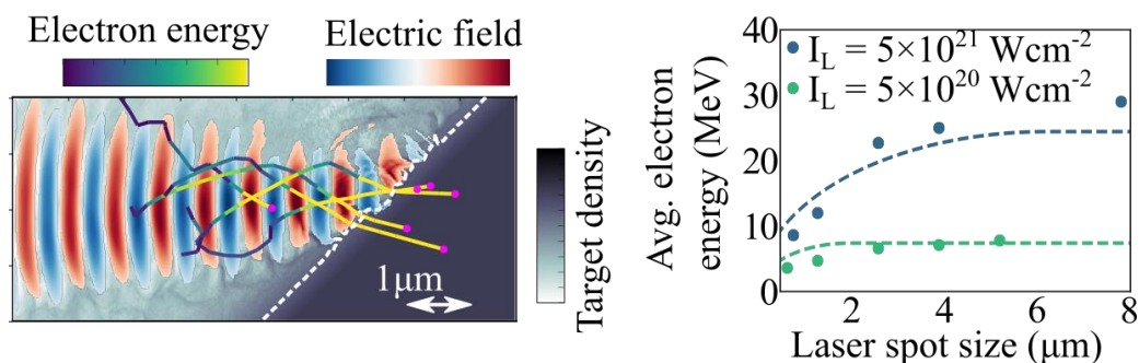
図4: シミュレーション結果 (左図) レーザーがターゲットと相互作用する場所を拡大して表示。レーザーがターゲットの表面で反射するポイントにおいて、レーザーから電子へエネルギーが効率的に与えられる(白い点線で表示された場所)。(右図) レーザーの集光サイズと強度に依存する電子の平均エネルギー。点線は、我々が導き出した新しい理論による予想。非常によく合っていることが分かる。
