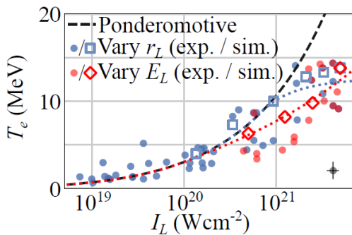
図 3：レーザーの強度を変化させて、電子のエネルギーをプロットした図。赤と青のデータ点はそれぞれ、(a) レーザーのエネルギーを変化させて、レーザーの強度を変化させた場合、(b) レーザーのエネルギーは一定で、レーザーの集光サイズを変化させることで、レーザーの強度を変化させた場合、に相当する。◇及び□は、スーパーコンピューターを用いて計算した結果を示す。黒い点線は、従来の理論の予想を示すが、どちらの結果も、レーザーの集光強度が 10^{21} W/cm 2 を超える領域で従来の理論の予測からずれることを示している。
